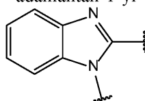
benzoimidazol-1,2-yl
