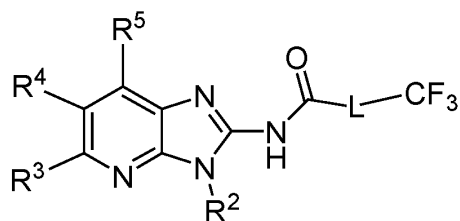
Formula A-36
