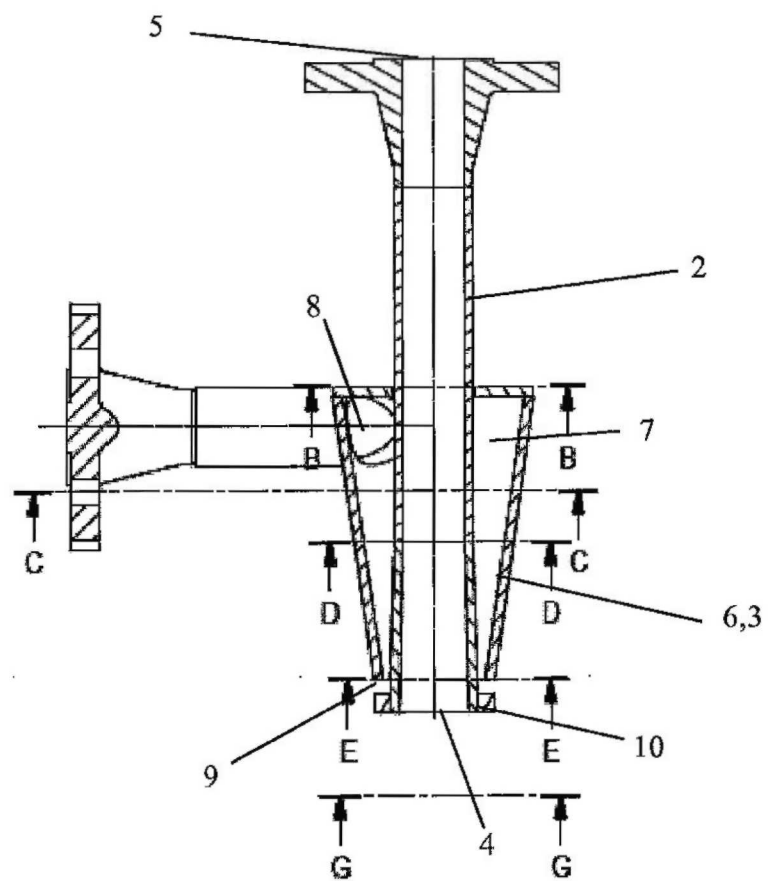
Fig. 3 Section A-A
