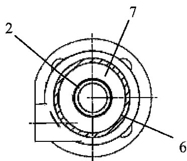
Fig. 6 Section D-D
