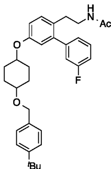
N -(2-(5-((4-((tert-butyl)benzyl)oxy)cyclohexyl)oxy)-3'-fluoro-[1,1'-biphenyl]-2-yl)ethyl)acetamide (63)
