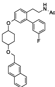
N -(2-(3'-fluoro-5-((4-(naphthalen-2-ylmethoxy)cyclohexyl)oxy)-[1,1'-biphenyl]-2-yl)ethyl)acetamide (67)
