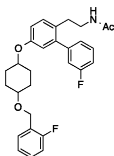
N -(2-(3'-fluoro-5-((4-((2-fluorobenzyl)oxy)cyclohexyl)oxy)-[1,1'-biphenyl]-2-yl)ethyl)acetamide ( 49 )
