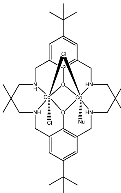
[L 1 Co 2 Cl 2 Nu]
