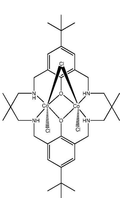
[L 1 Co 2 Cl 3 ] + [B-H] -
