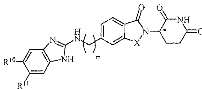
(V)
