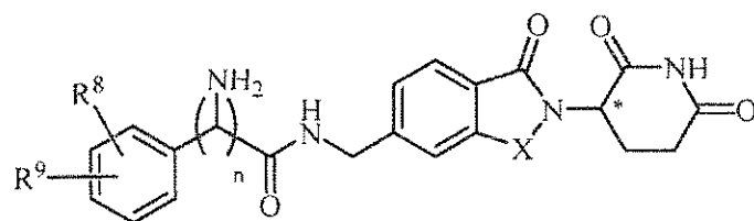
(IV)
