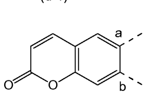
(d-6)
