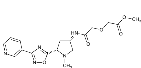
CAS 1396491-78-3,
