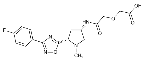
CAS 1212507-42-0.
