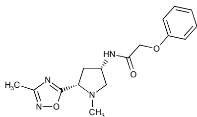
CAS 1212554-50-1,
