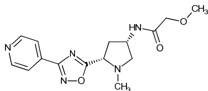
CAS 1212658-99-5,
