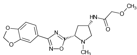
CAS 1212688-74-8,
