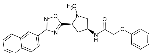
CAS 1212567-76-4,
