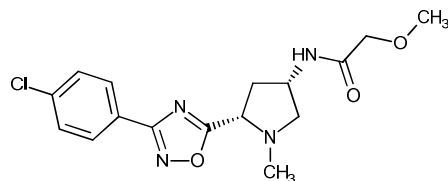
CAS 1212634-69-9,
