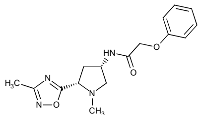
CAS 1212554-50-1,
