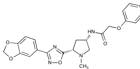
CAS 1212733-42-0,
