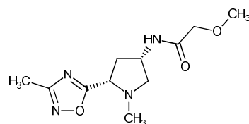
CAS 1212685-85-2,
