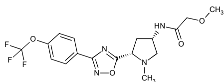
CAS 1212728-70-5,
