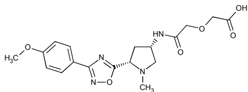
CAS 1212683-11-8,
