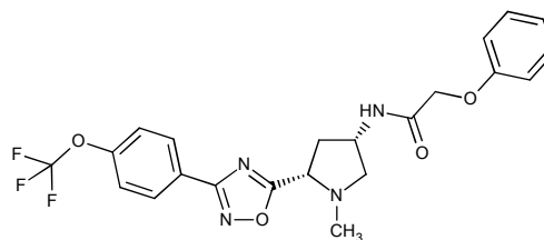
CAS 1212628-07-3,
