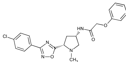
CAS 1212633-89-0,
