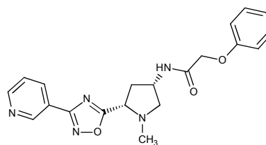
CAS 1212723-70-0,
