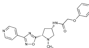
CAS 1212664-04-4,
