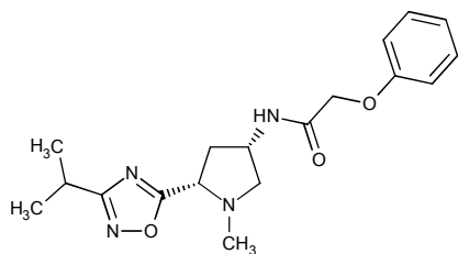
CAS 1212619-73-2,
