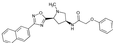
CAS 1212567-76-4,
