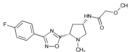
CAS 1212561-17-5,
