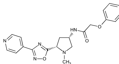
CAS 1212664-04-4,
