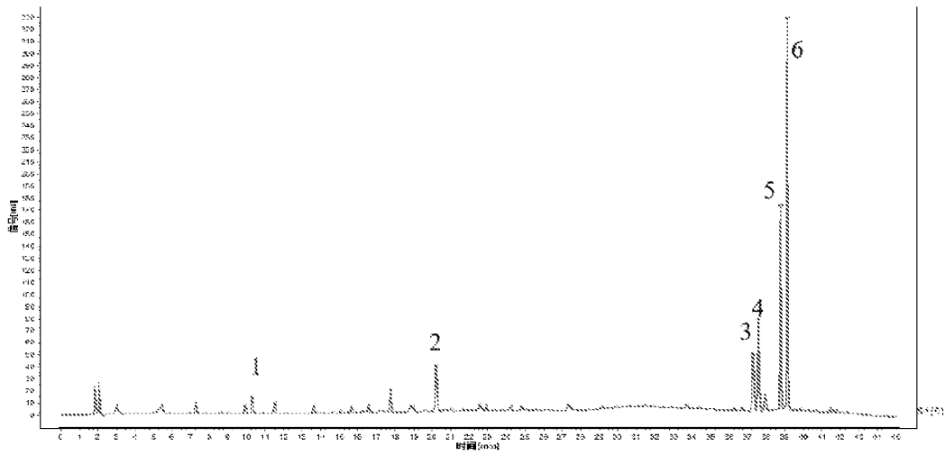
峰1：原儿茶酸
