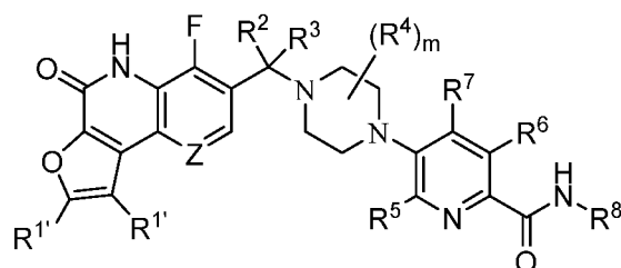
Formula (Im);
