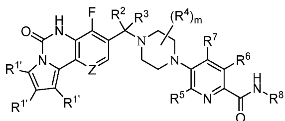
Formula (Ie);
