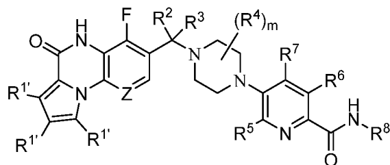
Formula (Ia);
