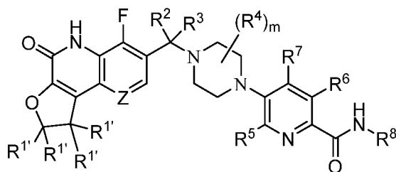
Formula (Io);
