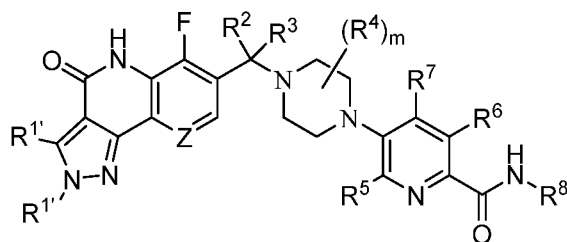
Formula (Ik);
