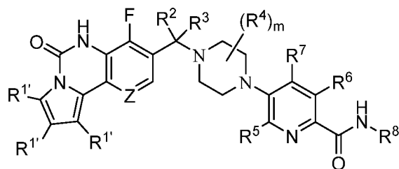
Formula (Ie);
