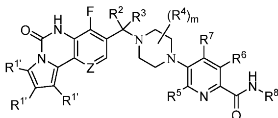
Formula (Ie);
