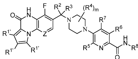
Formula (Ia);
