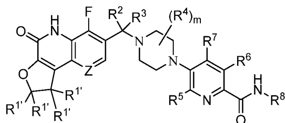
Formula (Io);
