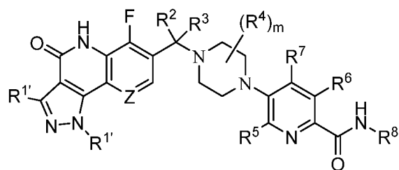
Formula (Il);
