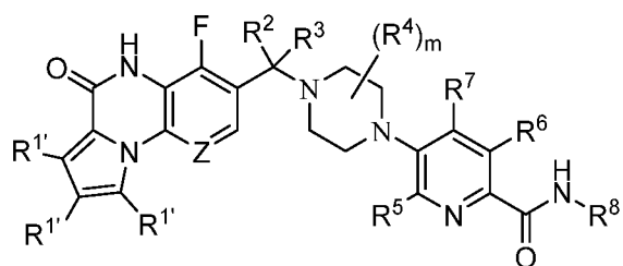
Formula (Ia);
