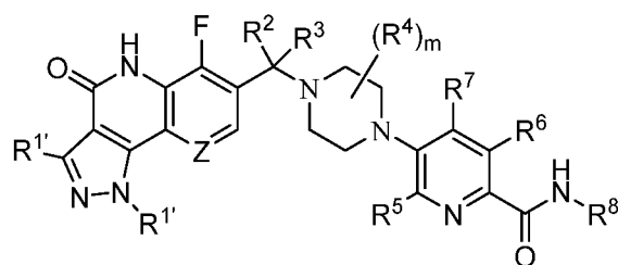
Formula (Il);
